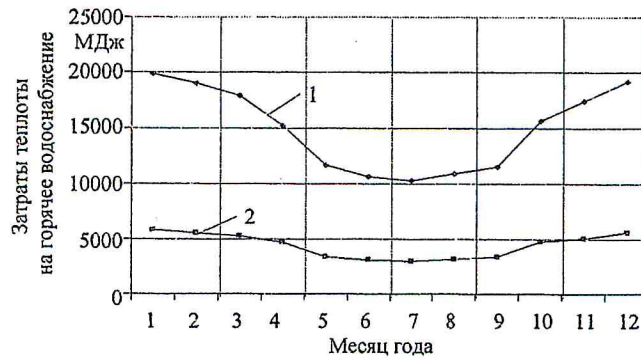
Рис. 3. Графики тепловых характеристик по месяцам для варианта 1: 1 – среднемесячная потребность теплоты на горячее водоснабжение по месяцам; 2 – среднемесячная теплота, утилизированная утилизатором сточных вод
