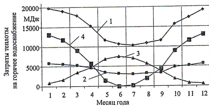
Рис. 4. Графики тепловых характеристик по месяцам для варианта 2: 1 – среднемесячная потребность теплоты на горячее водоснабжение по месяцам; 2 – среднемесячная теплота, утилизируемая утилизатором сточных вод; 3 – среднемесячная теплота, вырабатываемая солнечным коллектором; 4 – вспомогательный график выбора площади солнечного коллектора из расчета полной компенсации затрат энергии в июле
