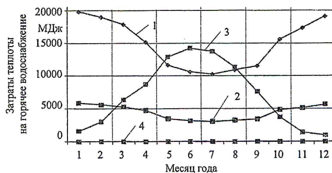
Рис. 6. Графики тепловых характеристик по месяцам для варианта 4:
